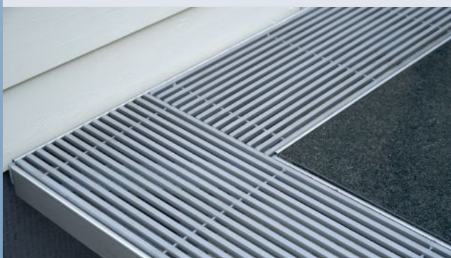
Rost QST 8x8
